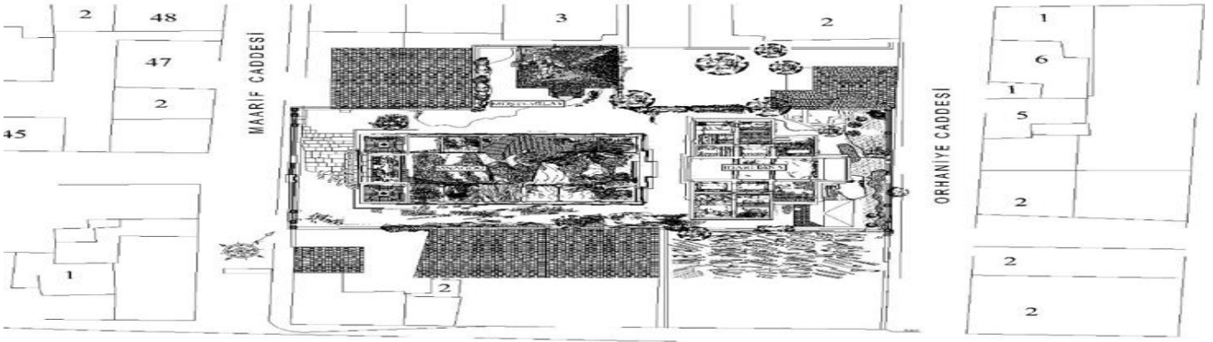
Şekil 3. Sinagog Kompleksi vaziyet planı (Kaynak: Vakıflar Bölge Müdürlüğü, 2007)
